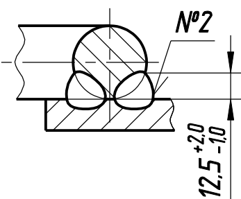
А-А (1:1) 2 места
