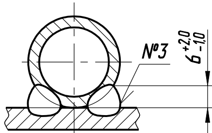
Б (1:1) 4 места
